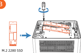
M.2 2280 SSD
